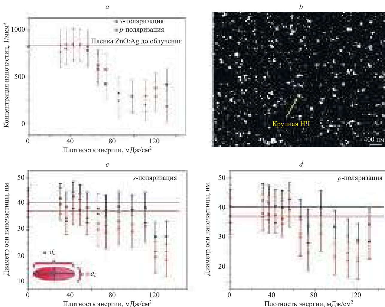
Рис. 7. Полученные из анализа СЭМ-снимков данные концентрации ( a ) и размера ( c , d ) наночастиц Ag в зависимости от плотности энергии в режимах s - ( a , c ) и p -поляризации ( a , d ), контрастное изображение СЭМ-снимка пленки после лазерного воздействия с плотностью энергии 121 мДж/см 2 ( b )
