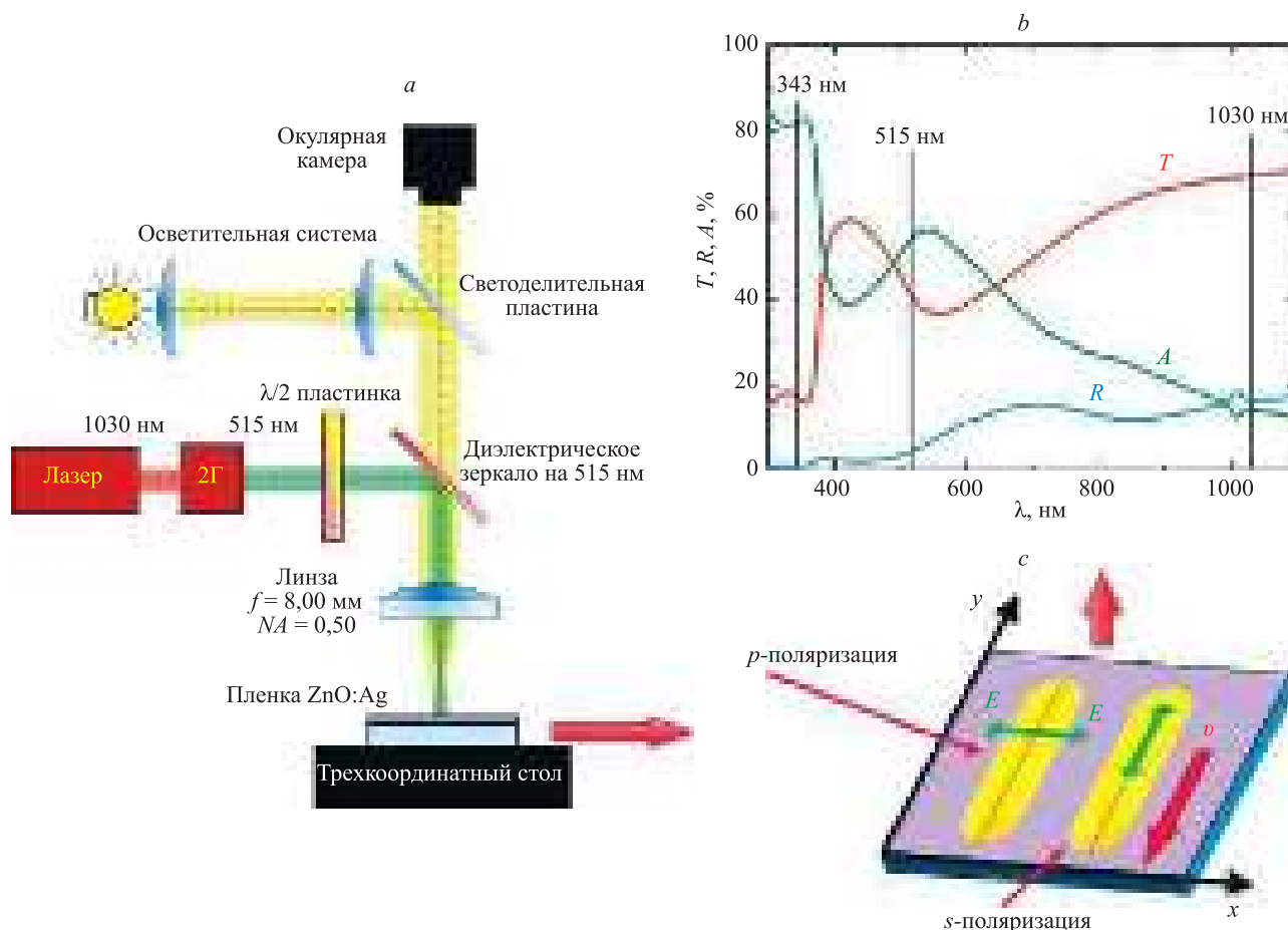
Рис. 1. Экспериментальная установка ( a ); спектральные характеристики пленки ZnO:Ag ( b ); ориентация вектора поляризации фемтосекундного излучения относительно направления сканирования ( c )
